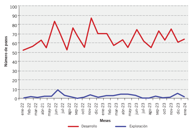
Pozos perforados
